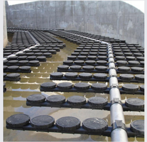
Difusores de Sistema Circular
