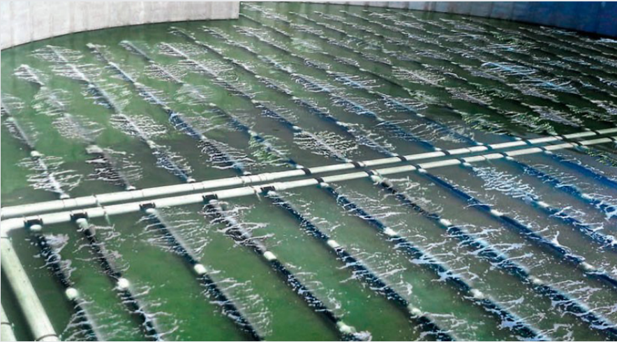
Difusores de Sistema Tubular
